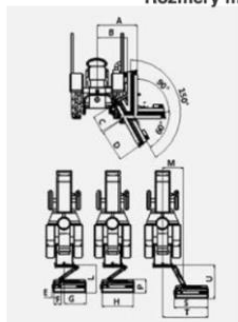
Rozmery mulčovačov v rôznych pracovných polohách
