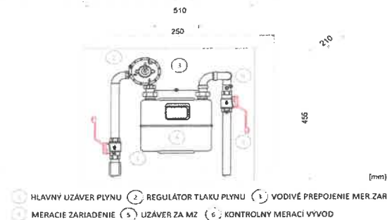
Detail meracej (domovej) regulačnej zostavy
