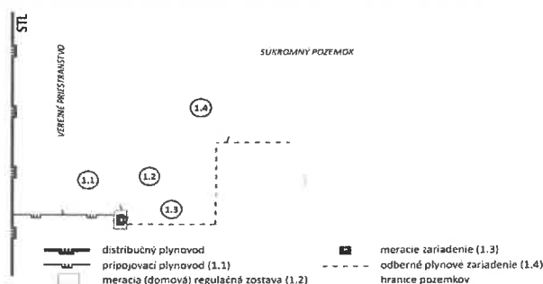
Orientačný náčrt zariadení podľa vyššie uvedenej špecifikácie
